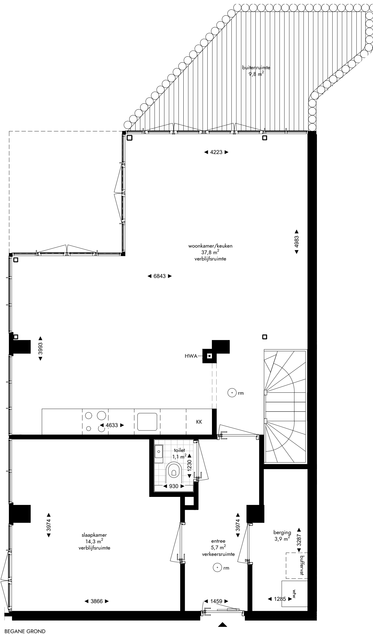
BEGANE GROND
