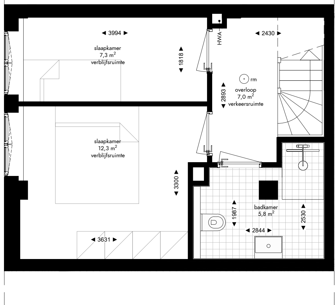
SOUTERRAIN
